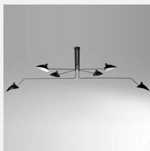
OGS-LD245-6 D2800*H700mm E14*6
