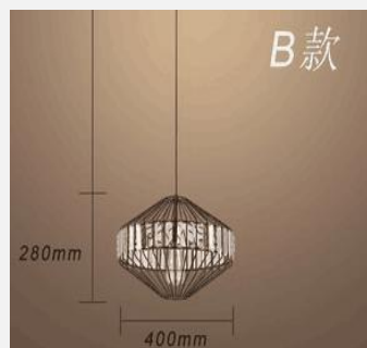
OGS-LD256B D400*H280mm E27*1
